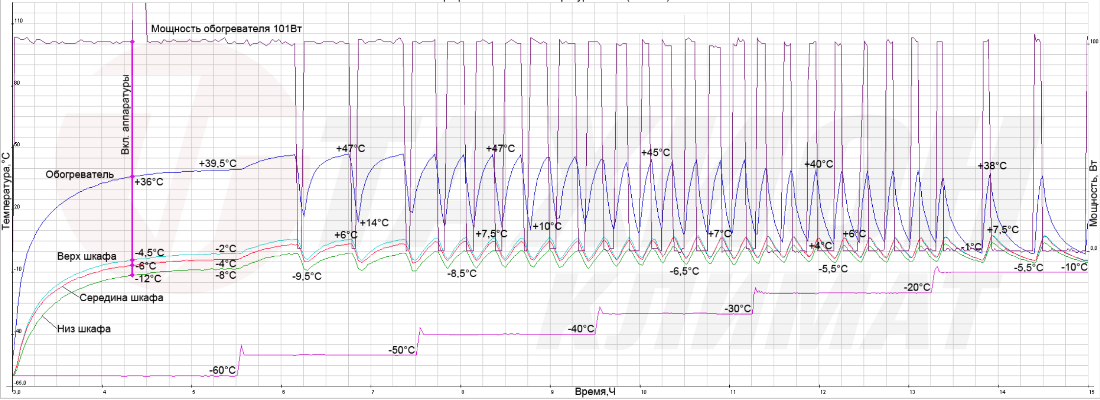
График изменения температуры ТШ-3 (с БУК-4)
