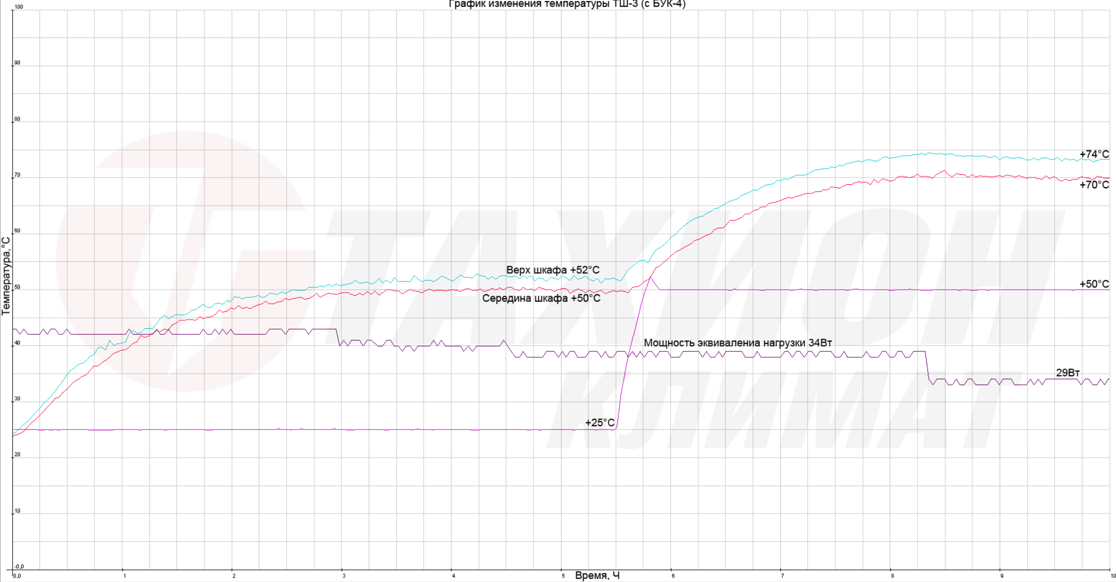
График изменения температуры ТШ-3 (с БУК-4)
