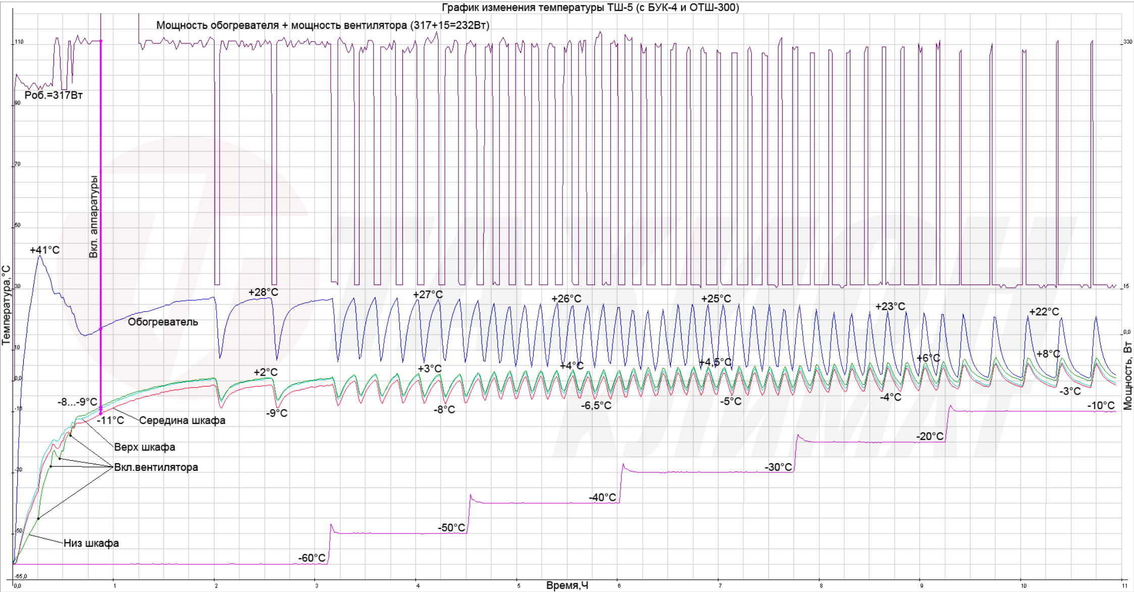
График изменения температуры ТШ-5 (с БУК-4 и ОТШ-300)
