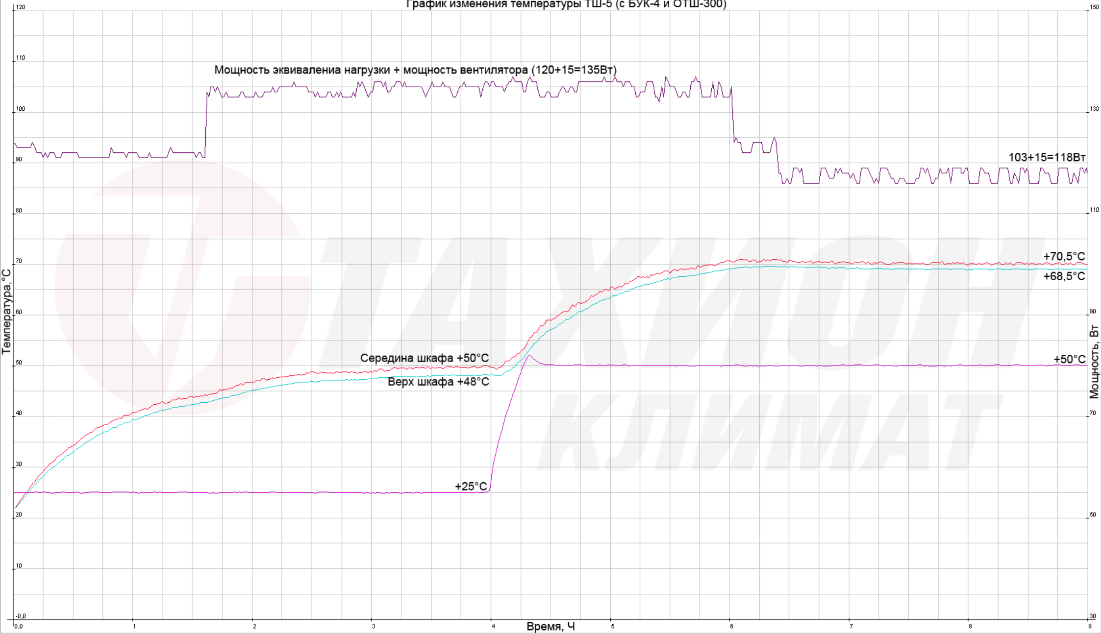
График изменения температуры ТШ-5 (с БУК-4 и ОТШ-300)
