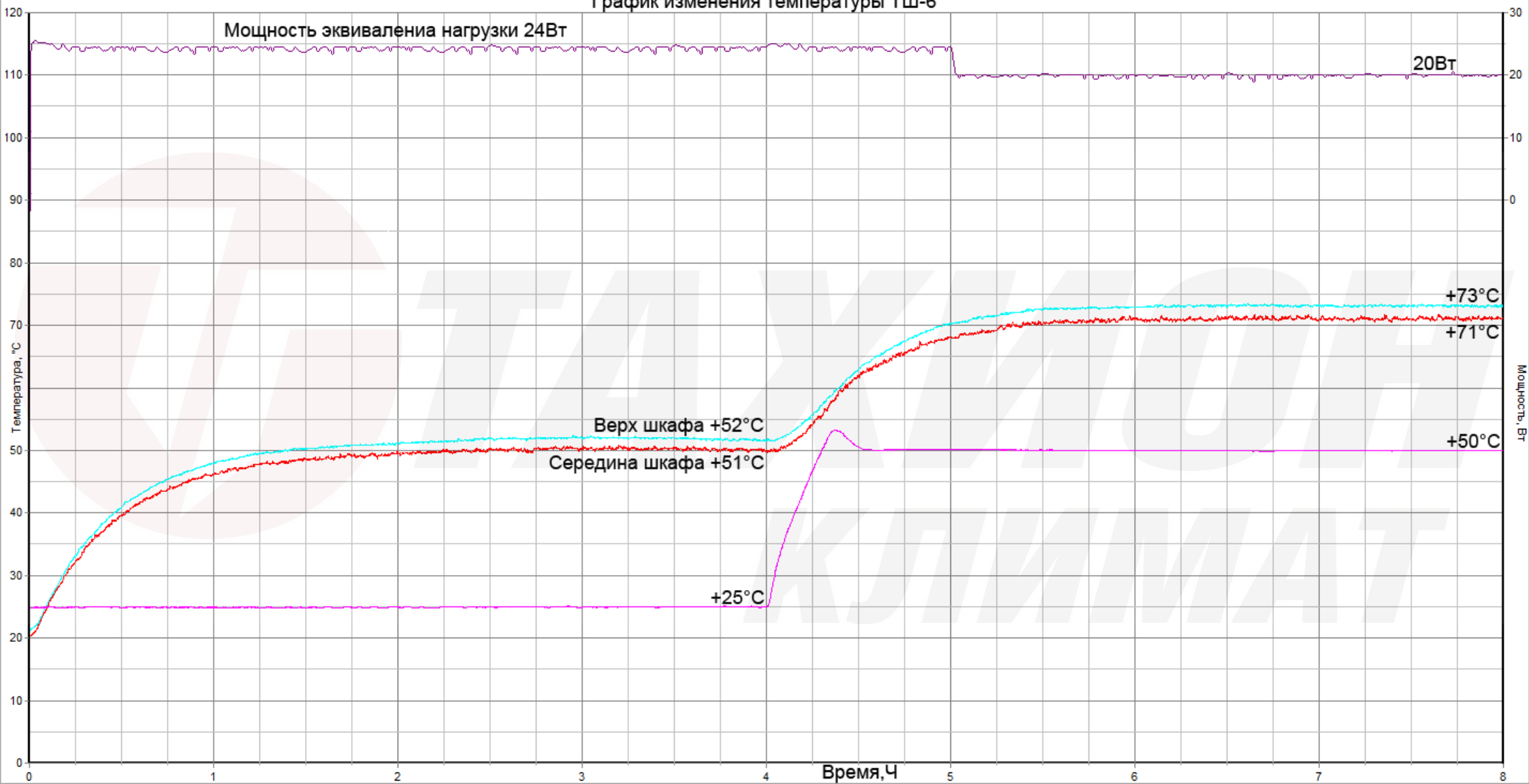
График изменения температуры ТШ-6
