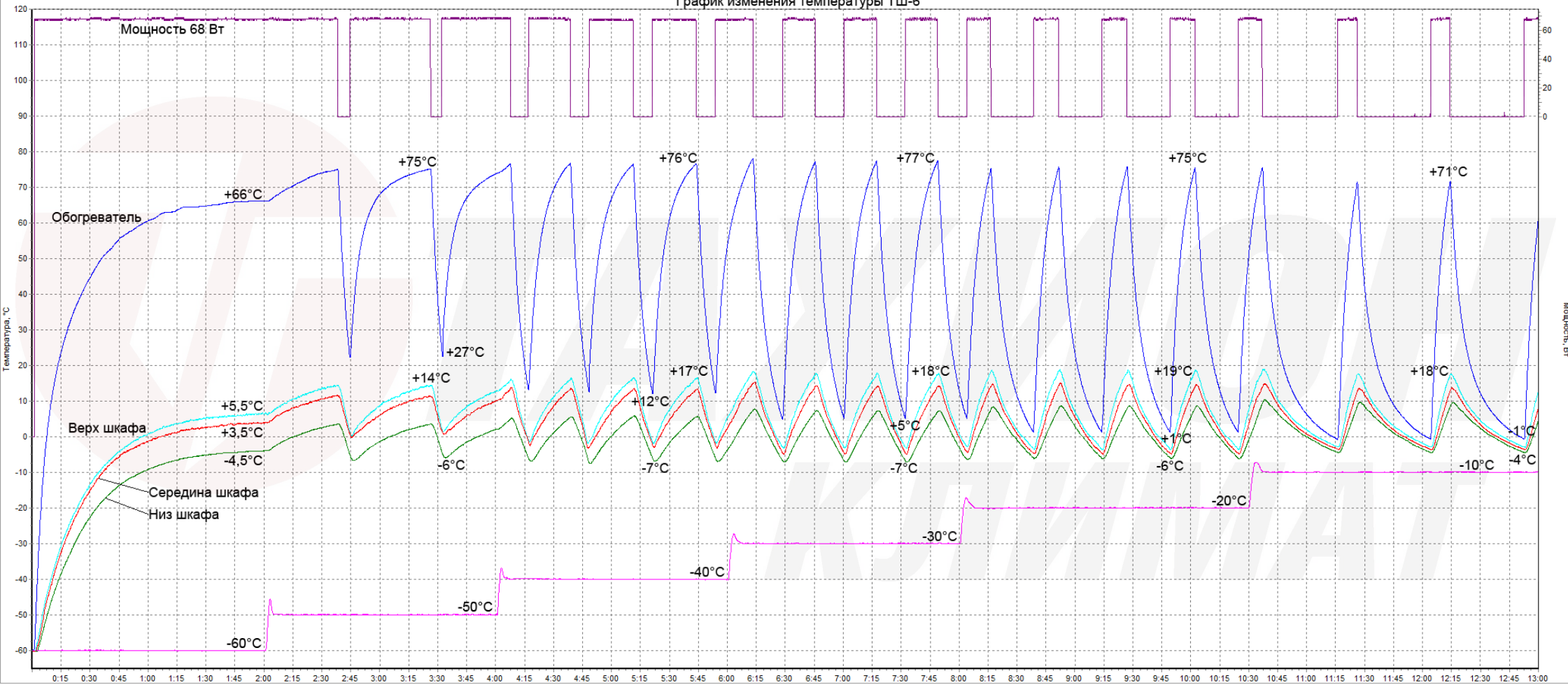
График изменения температуры ТШ-6
