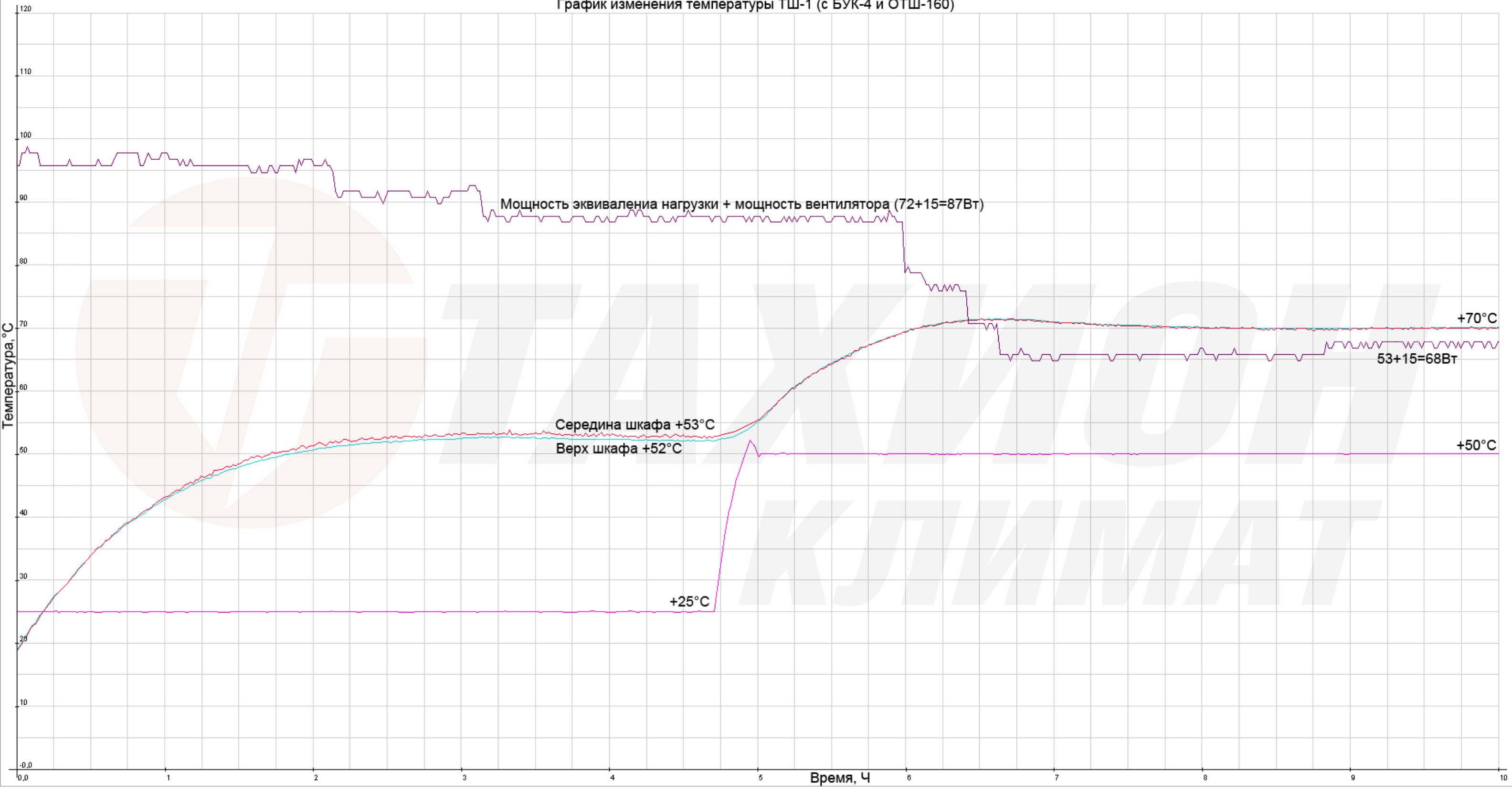
График изменения температуры ТШ-1 (с БУК-4 и ОТШ-160)
