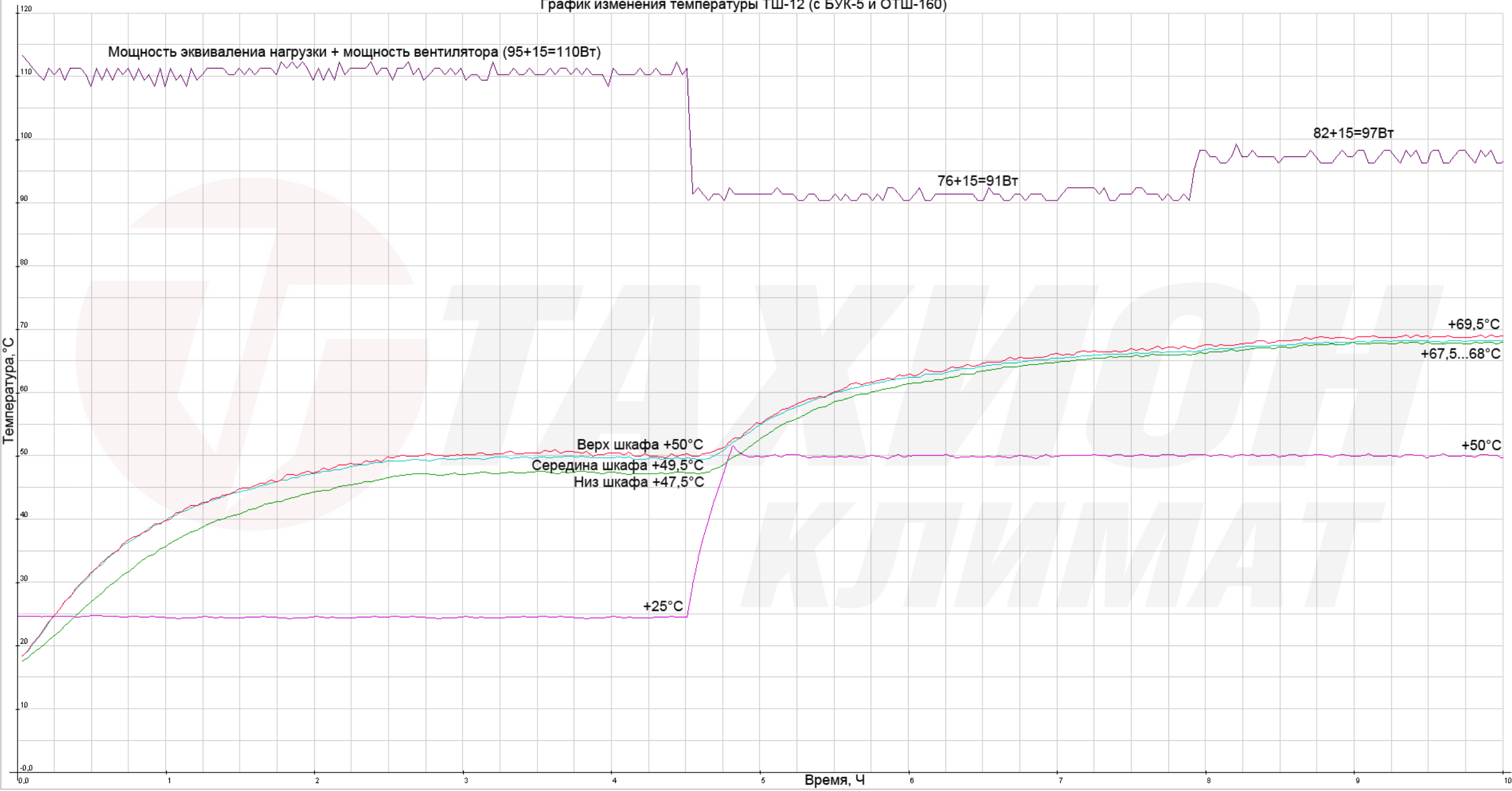
График изменения температуры ТШ-12 (с БУК-5 и ОТШ-160)
