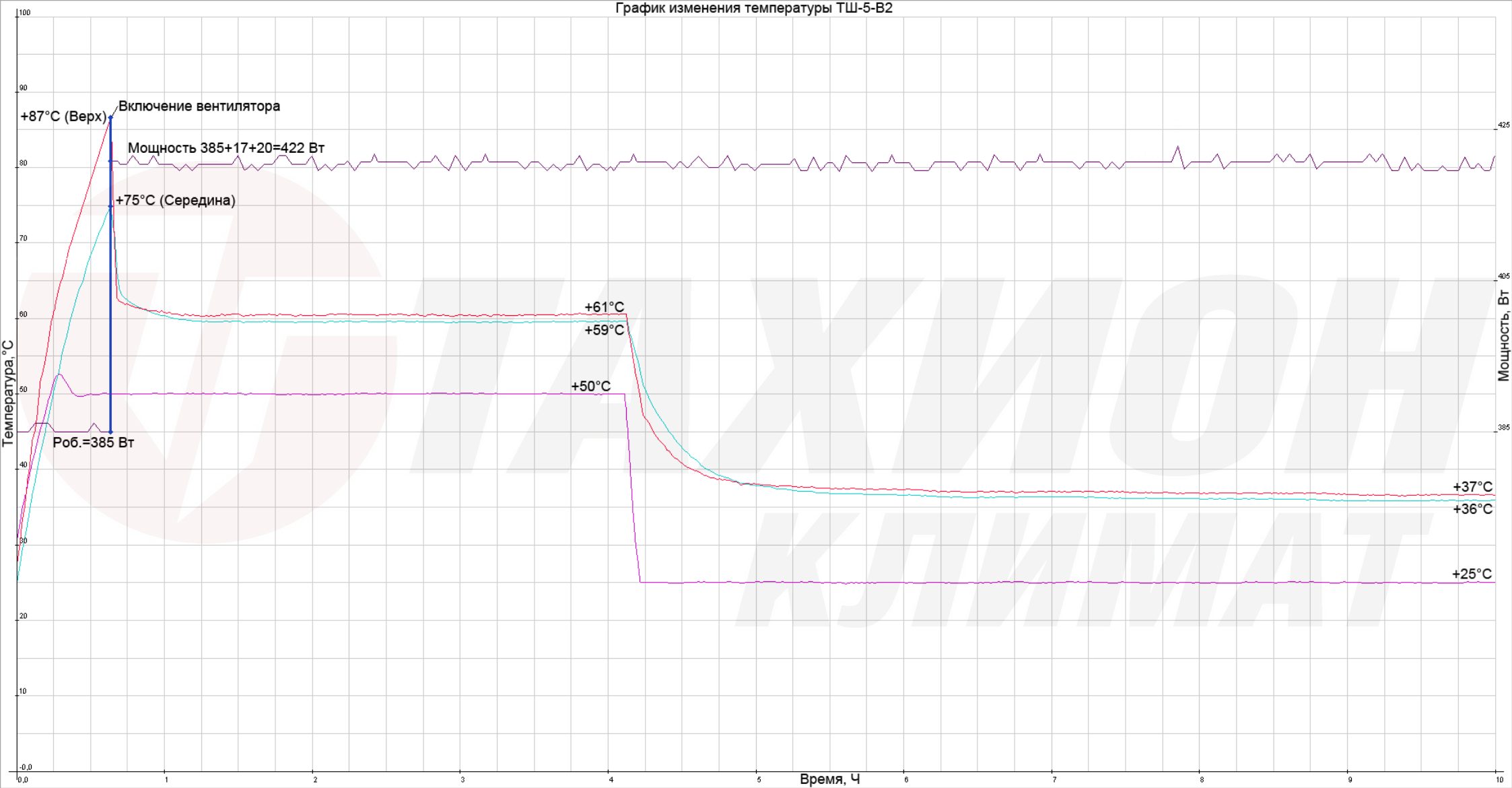
График изменения температуры ТШ-5-В2
