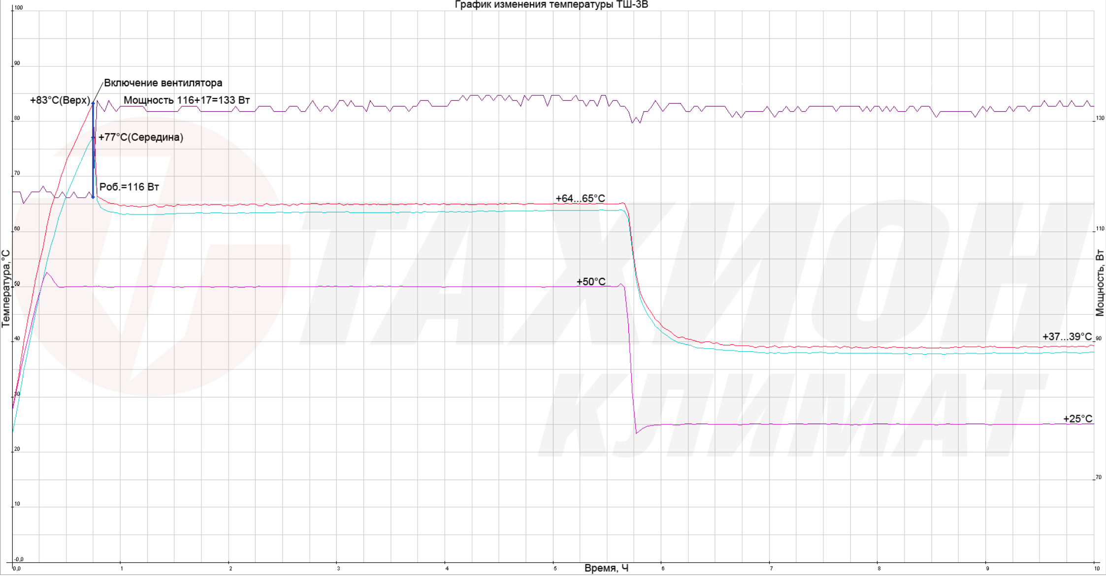
График изменения температуры ТШ-3В
