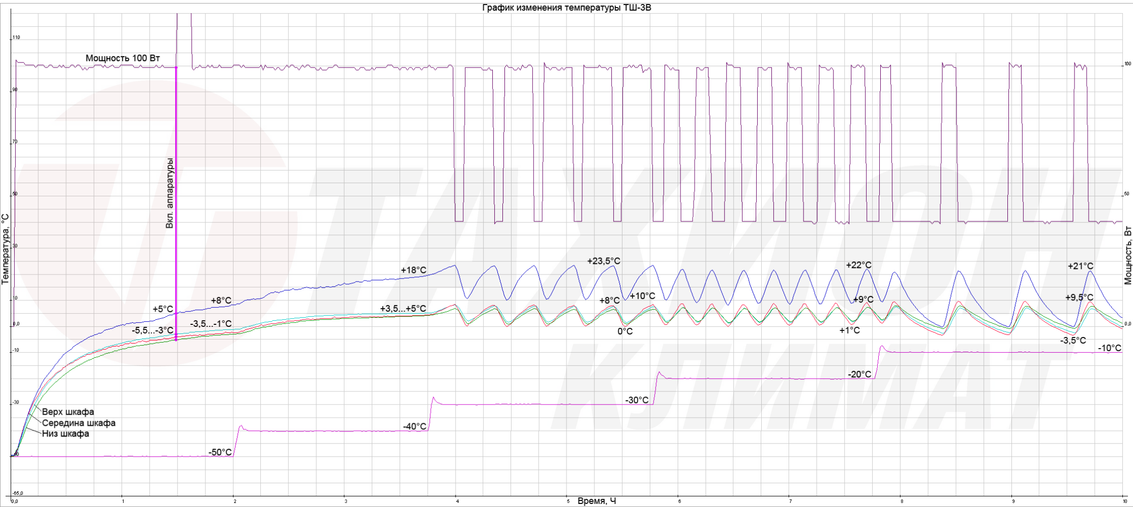
График изменения температуры ТШ-ЗВ
