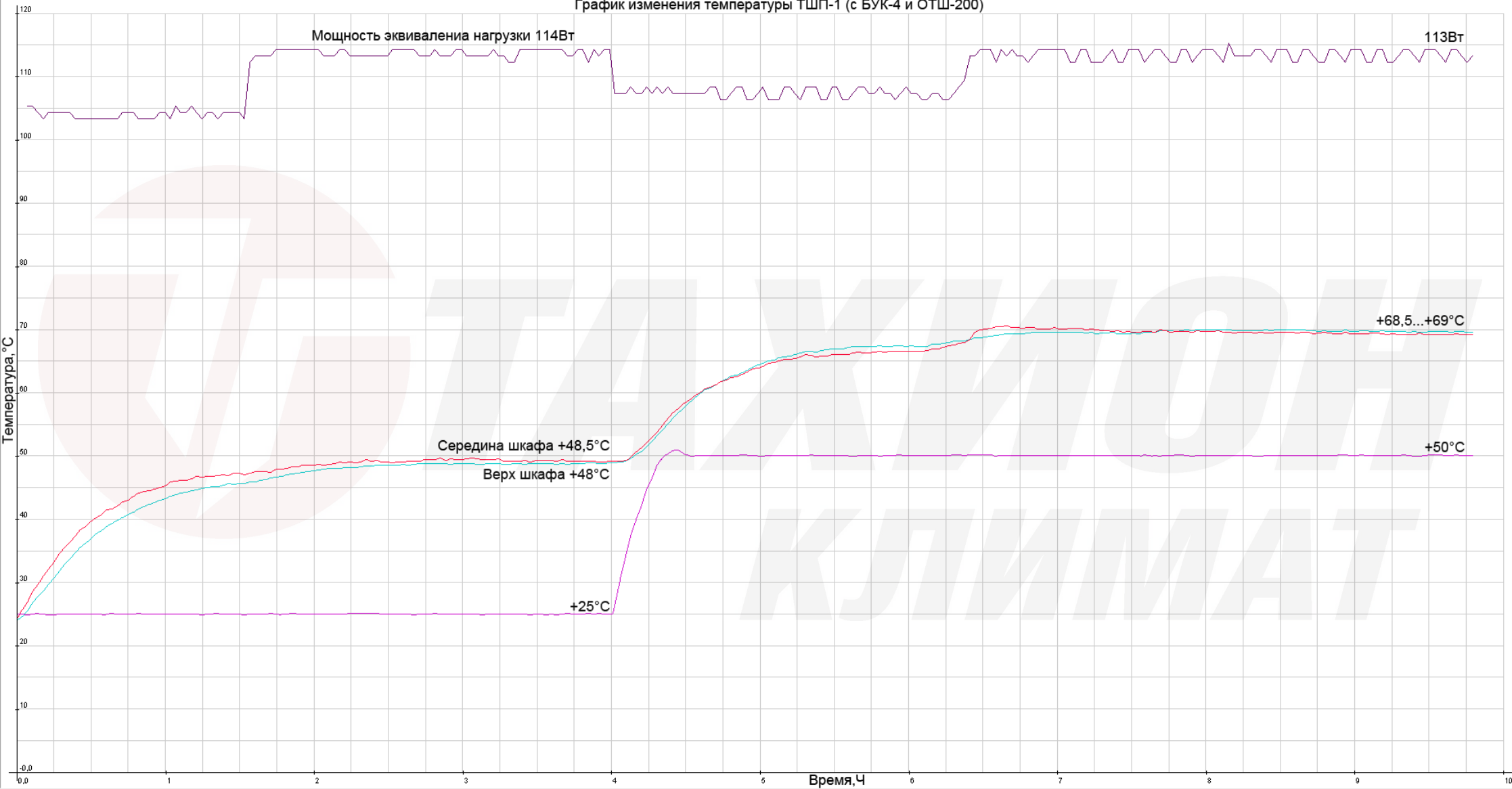
График изменения температуры ТШП-1 (с БУК-4 и ОТШ-200)
