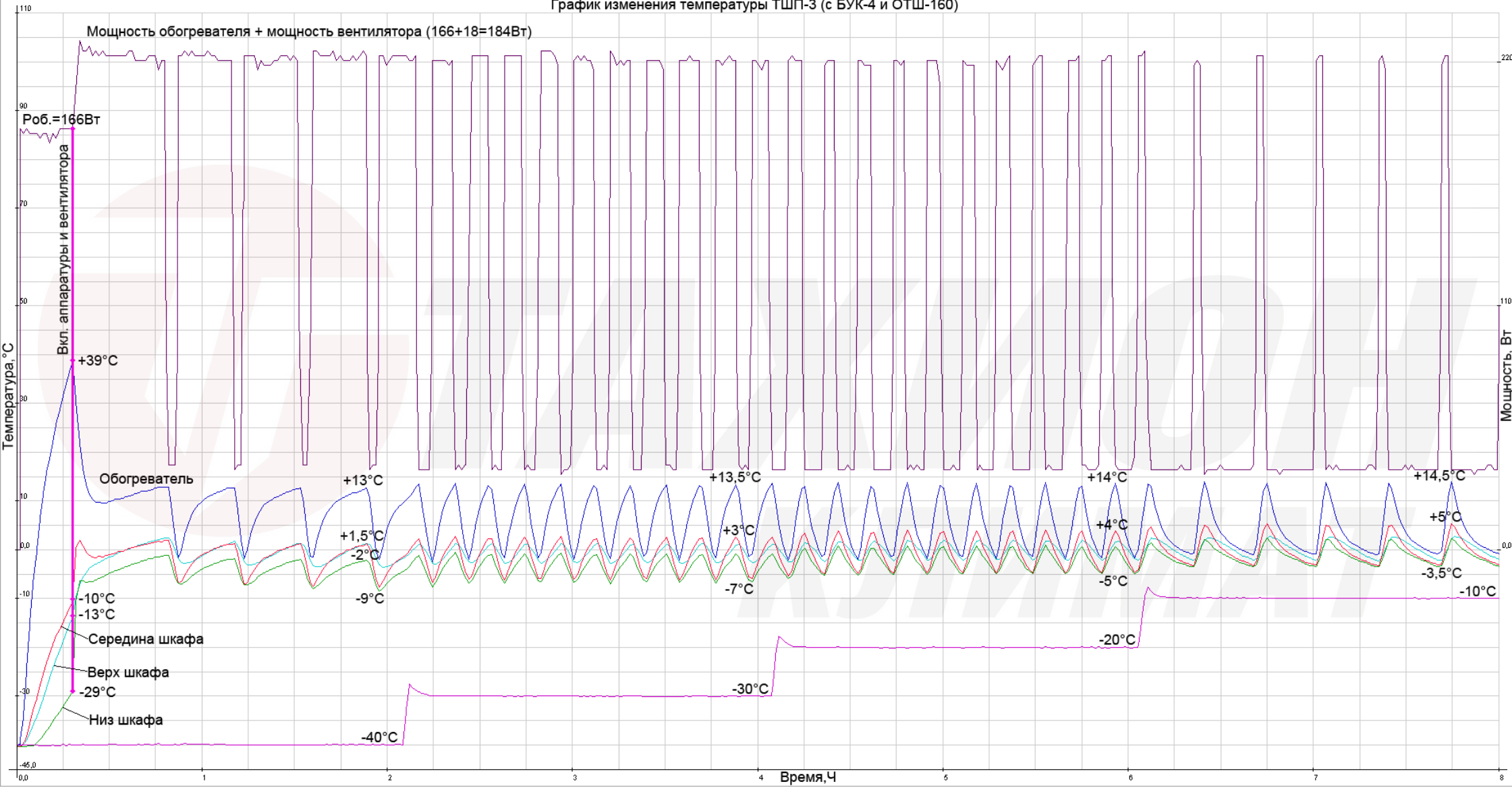
График изменения температуры ТШП-3 (с БУК-4 и ОТШ-160)
