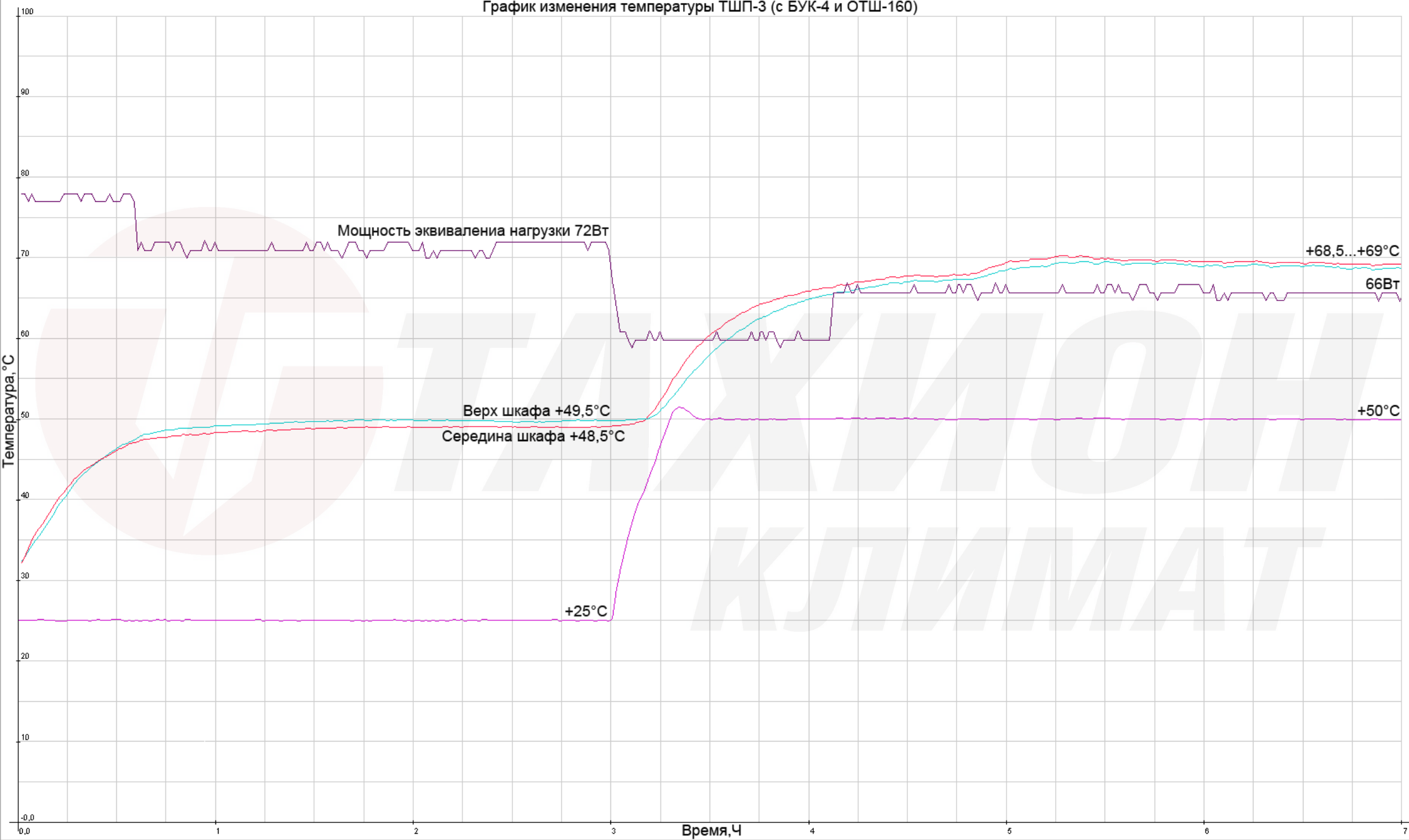
График изменения температуры ТШП-3 (с БУК-4 и ОТШ-160)
