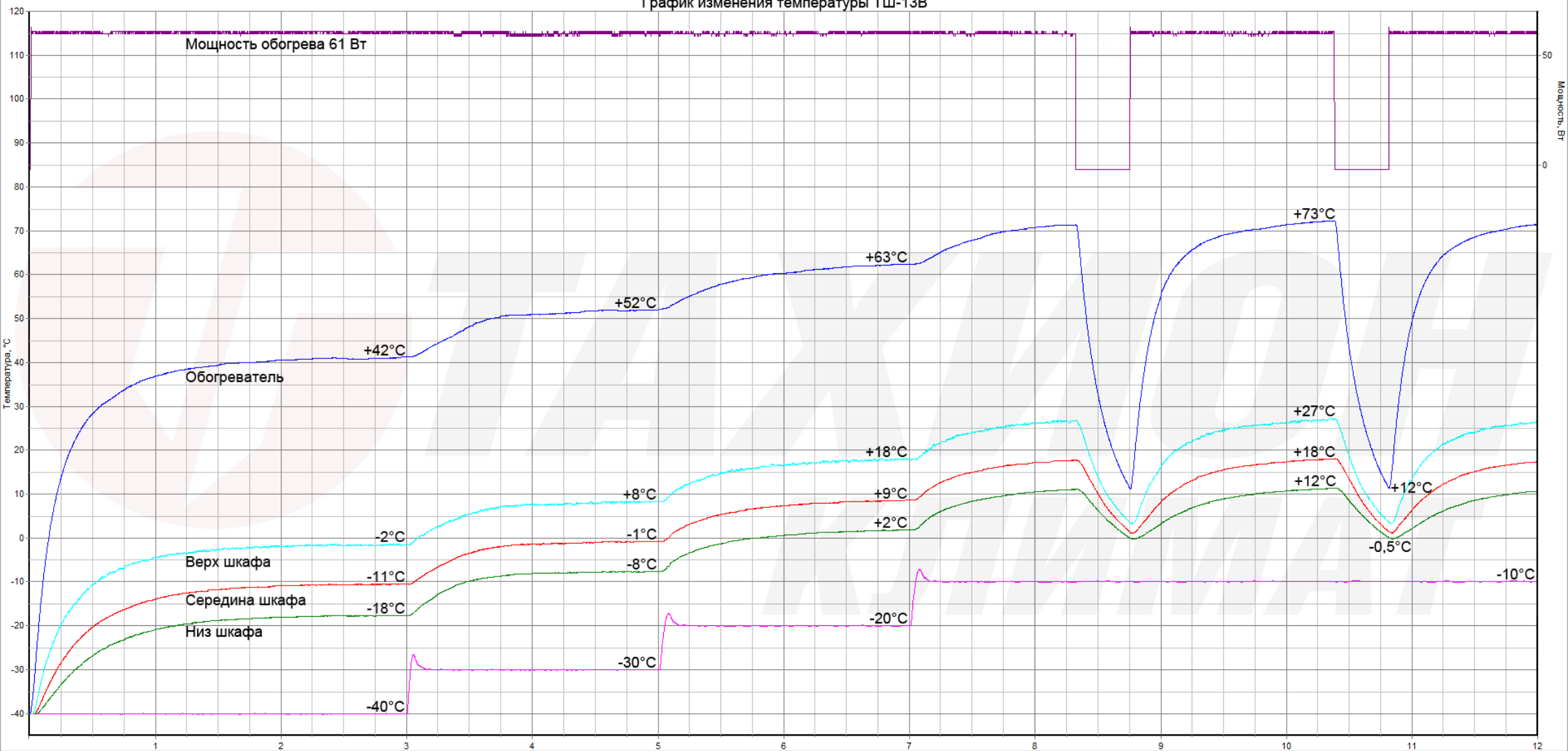
График изменения температуры ТШ-13В
